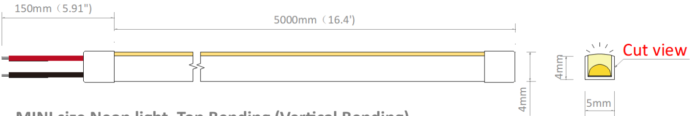
MINI size Neon light, Top Bending (Vertical Bending)
