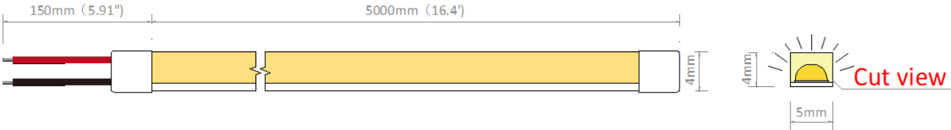
MINI size Neon light, Top Bending (Vertical Bending)
